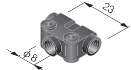
M6 tee P/N 9738 POM M6 Quantity: 1
